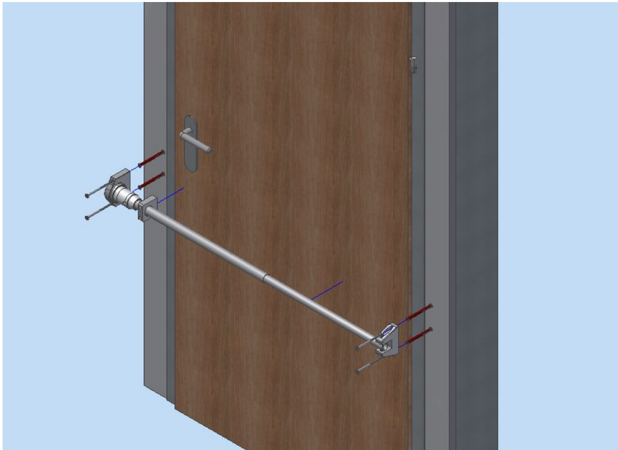
Montagebeispiel
