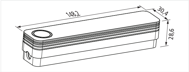
Abb. 12: Maßzeichnung
